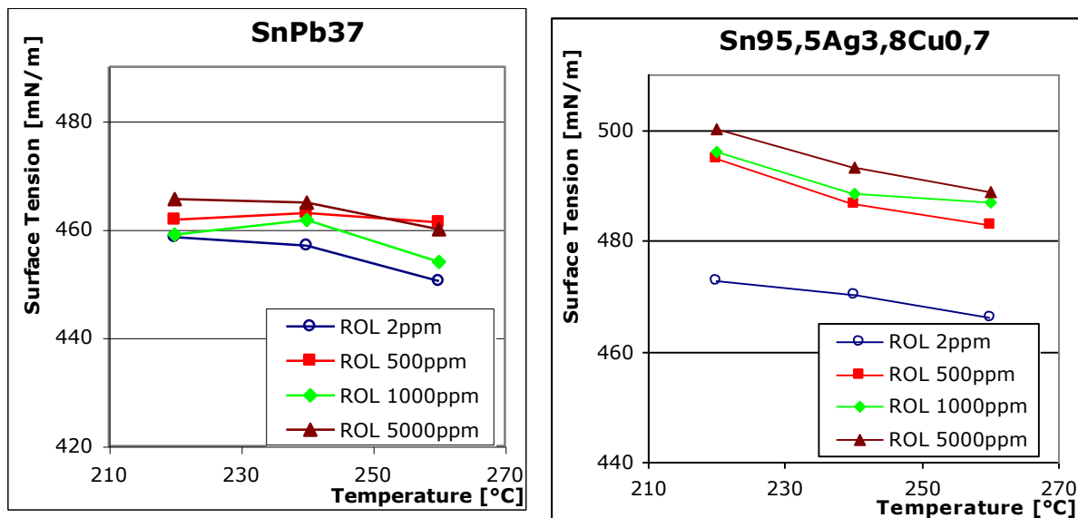
2. ábra: Felületi feszültség változása ólomtartalmú és ólommentes forrasztanyag esetén a hőmérséklet és maradék oxigén függvényében
