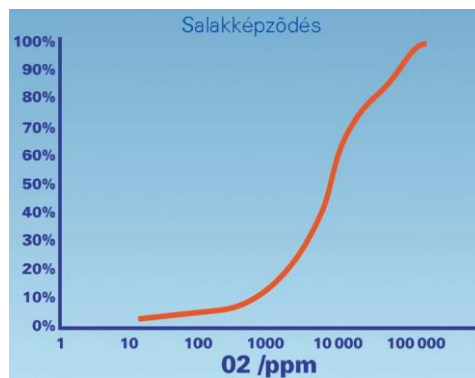
1. ábra: Salakképződés
