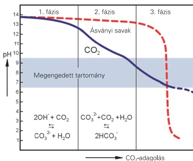
A \text{CO}_2 és ásványi savak semlegesítési görbéjének összehasonlítása
