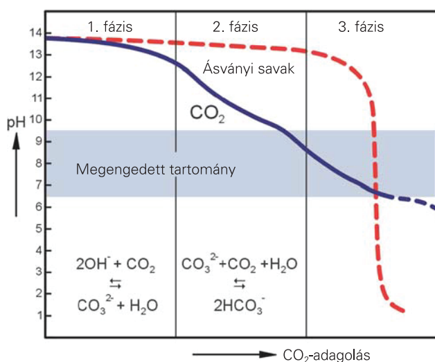
A CO 2 és ásványi savak semlegesítési görbéjének összehasonlítása
