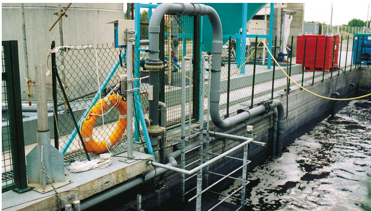
7. ábra: Lúgos szennyvíz semlegesítése szén-dioxiddal a textiliparban.
