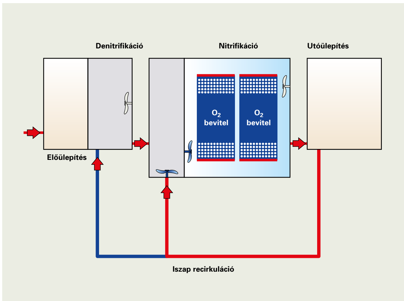
2. ábra. Egy szennyvíztisztító telep átalakítása Bior®-N eljárásra.
