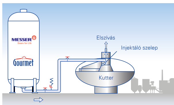
Kutterhűtés felső gázbeinjektálással
